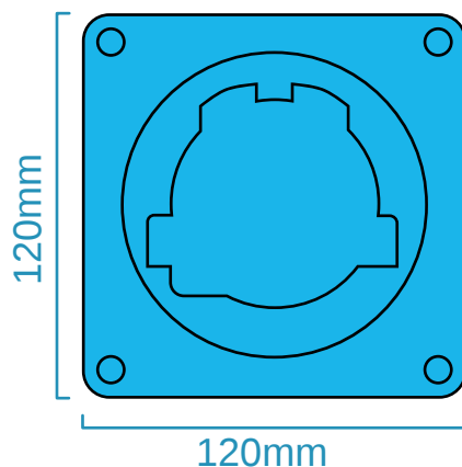
Ventilator mål set forfra
