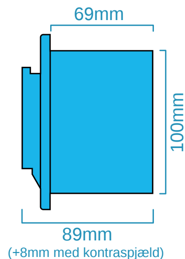
Ventilator mål set fra siden
